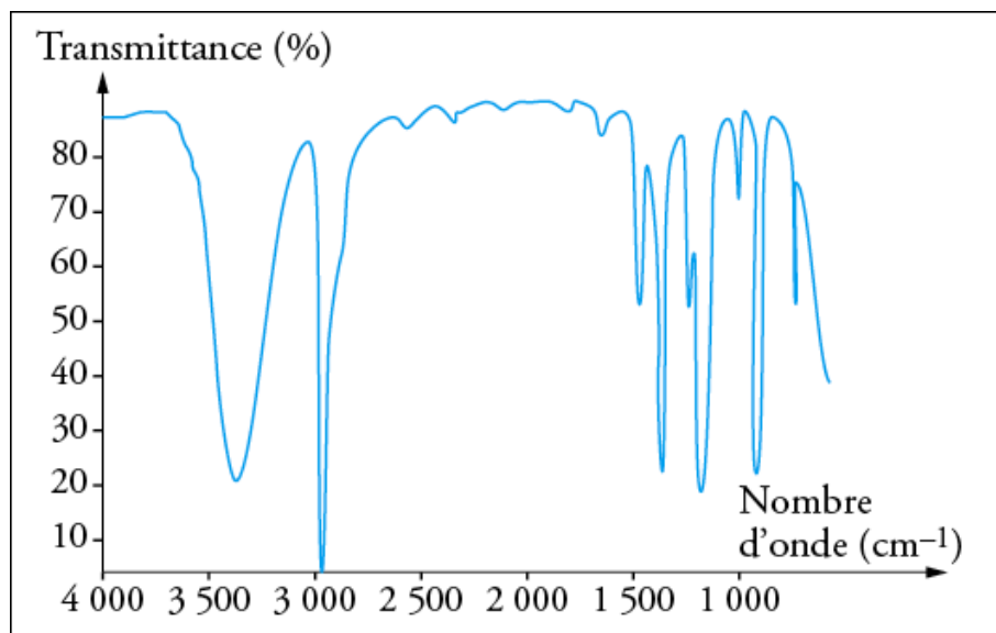
DOCUMENT 1 : SPECTRE IR DU PRODUIT OBTENU
