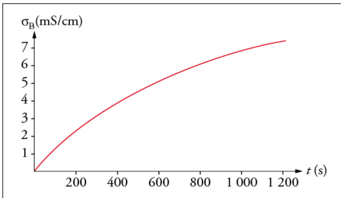
DOCUMENT 4 : ÉVOLUTION DE LA CONDUCTIVITÉ POUR L'EXPÉRIENCE B
