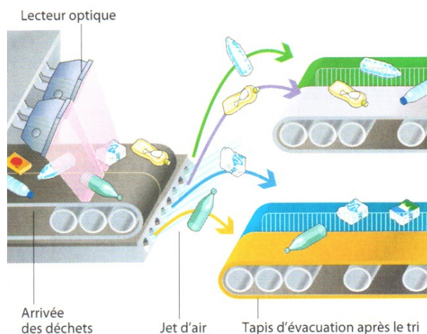
Trieur optique associé à une soufflerie
